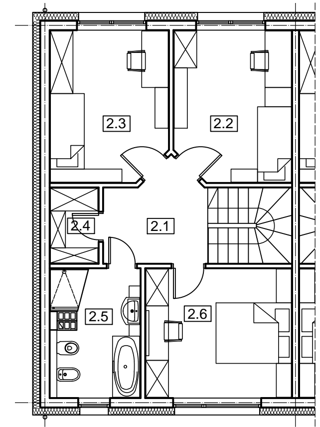
RZUT PIĘTRA
