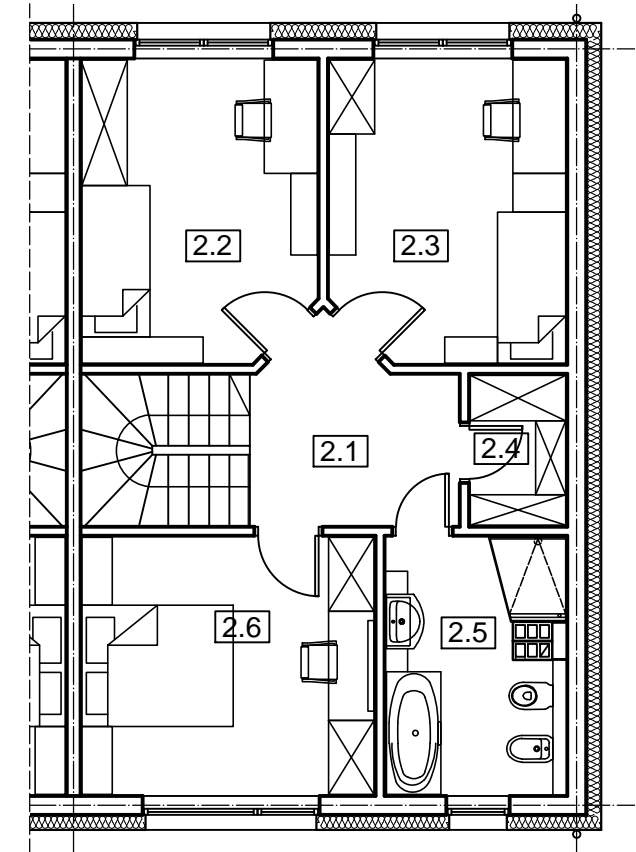
RZUT PIĘTRA
