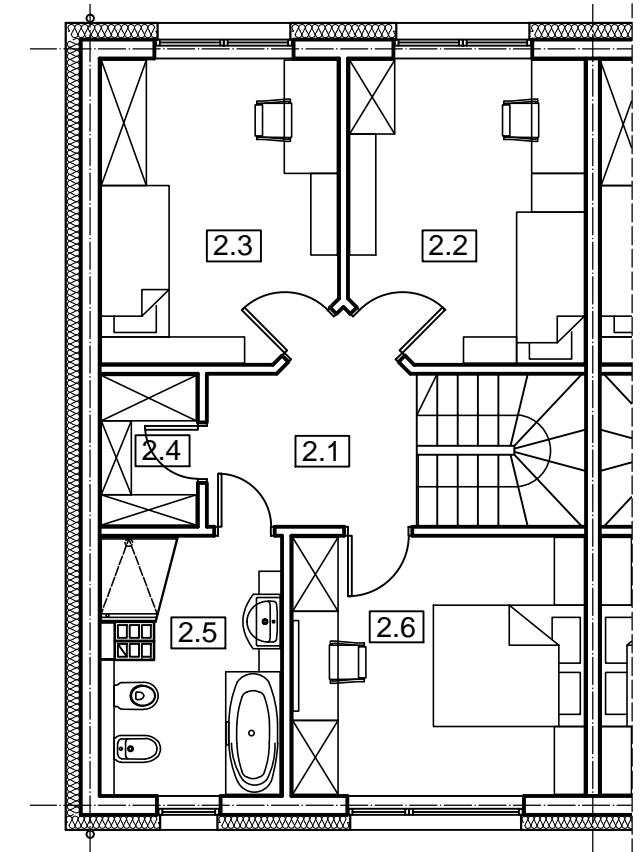
RZUT PIĘTRA
