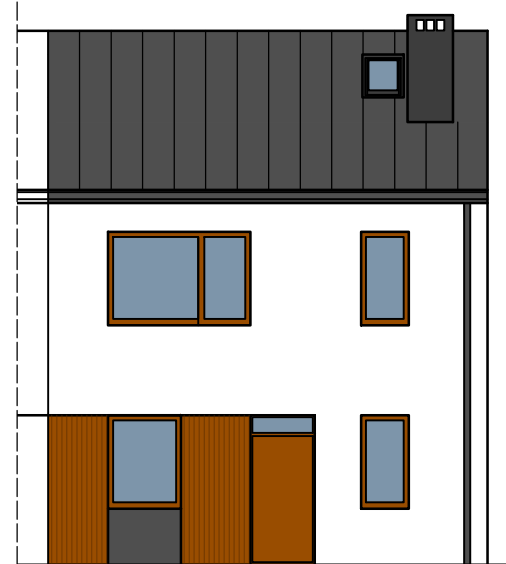
ELEWACJA WEJŚCIOWA
