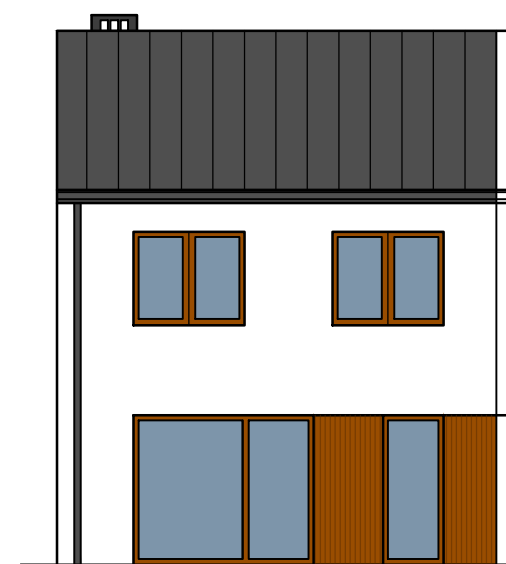
ELEWACJA OGRODOWA
