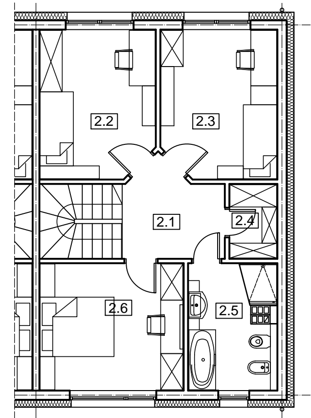
RZUT PIĘTRA
