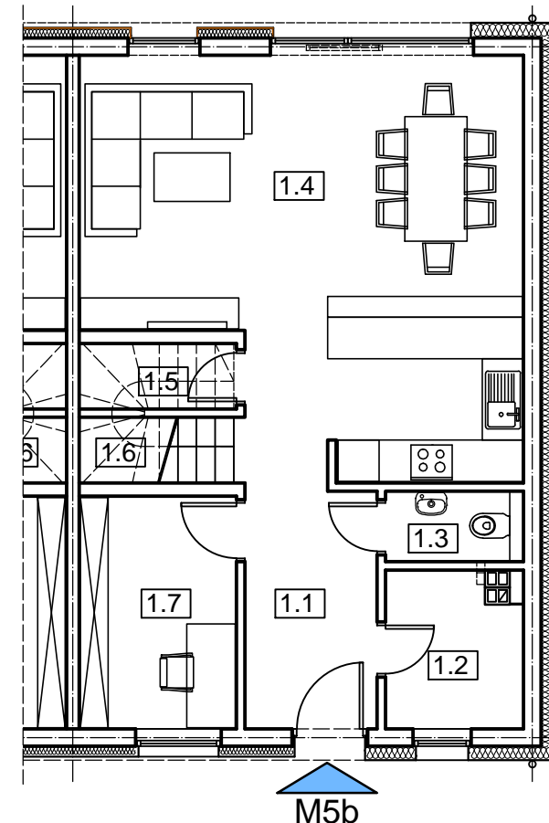
RZUT PARTERU
