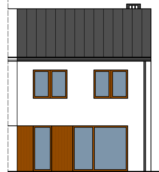
ELEWACJA OGRODOWA
